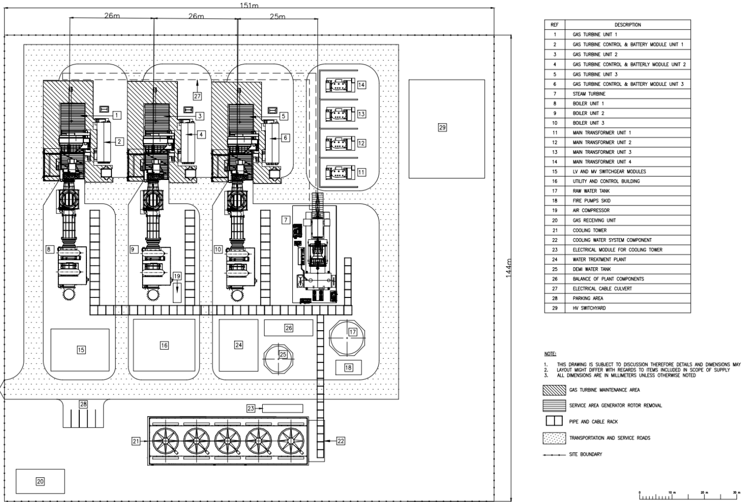
Рисунок 2. Орієнтовний компоновальний план станції.
